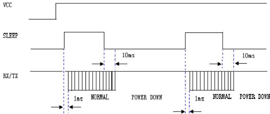
图 3: 休眠时序图
